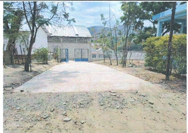
Foto 4: MEJORAMIENTO DE LOSA DE PATIO EN EL AREA DE INGRESO AL PLANTEL, FINALIZADO
